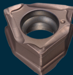
Plăcuță de tip XNMU06
